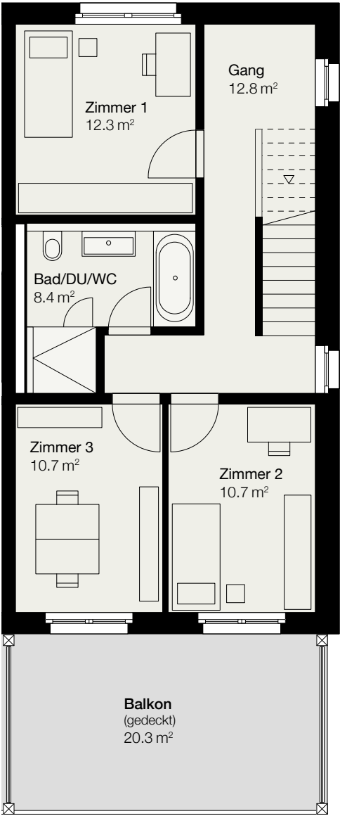
Obergeschoss
