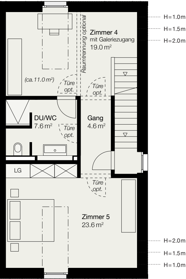
Dachgeschoss
